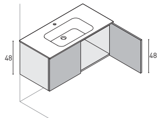
Waschtisch-Unterschrank mit 2 Türen.
