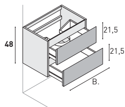
Waschtisch-Unterschrank mit 2 Auszügen.
