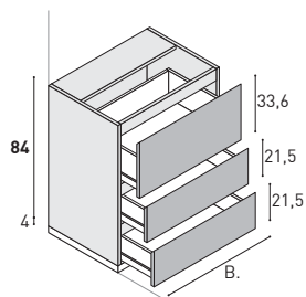
Unterschränk mit 3 Auszügen.
