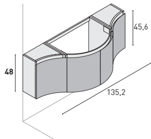
Waschtisch-Unterschrank gerundet mit 4 Türen.
