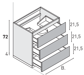
Waschtisch-Unterschrank mit 3 Auszügen.
