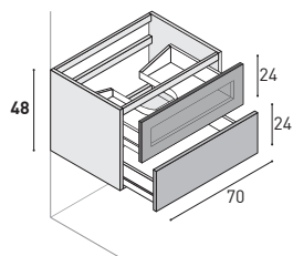
Waschtisch-Unterschrank mit 1 Obere-Auszug mit schwarzem Aluminiumrahmen + Stop-sol-Glas, 1 Untere-Auszug. Glasfront nur mit PROFILO-Griff kompatibel. KEIN Push-Pull.
