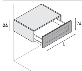
Unterschrank mit 1 Auszug mit schwarzem Aluminiumrahmen + Stop-sol-Glas. Glasfront nur mit PROFILO-Griff kompatibel. KEIN Push-Pull.
