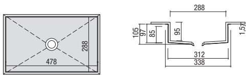
SIRIO HPS1 47,8 x 28,8 cm für Waschtisch-Unterschranke ≥ 60
