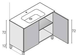
Waschtisch-Unterschrank mit 2 Türen, 1 Glas-Einlegeboden. Bodenstehend.
