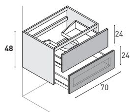
Waschtisch-Unterschrank mit 1 Obere-Auszug, 1 Untere-Auszug mit schwarzem Aluminiumrahmen + Stop-sol-Glas. Glasfront nur mit PROFILO-Griff kompatibel. KEIN Push-Pull.
