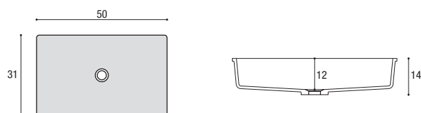
SMALL 50 x 31 cm für Waschtisch-Unterschranke \geq 60
