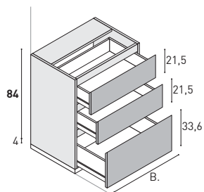
Unterschrank mit 3 Auszügen.
