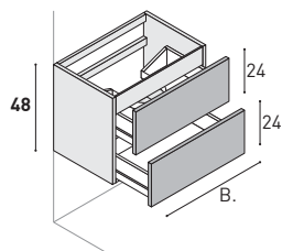
Waschtisch-Unterschrank mit 2 Auszügen.
