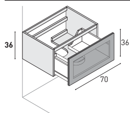
Waschtisch-Unterschrank mit 1 Auszug mit schwarzem Aluminiumrahmen + Stop-sol-Glas.
