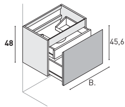
Waschtisch-Unterschrank mit 1 Auszug + 1 Schublade innen.
