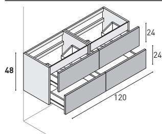
Waschtisch-Unterschrank für Doppel-Waschtisch mit 4 Auszügen.
