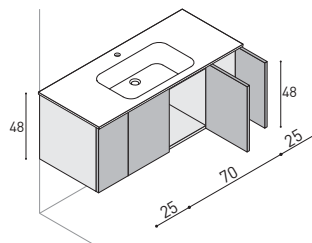
Waschtisch-Unterschrank mit 4 Türen, mit je 2 seitlichen Einlegeböden.
