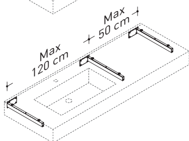
Gesamtbreite über 120 cm: Zusätzlich 1 weitere Halterung pro bis zu 50 cm Mehrbreite
