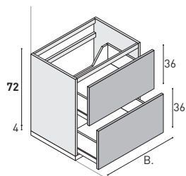
Waschtisch-Unterschrank mit 2 Auszügen. Geeignet NUR mit Waschtisch SLIM.
