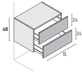
Unterschrank mit 2 Auszügen.
