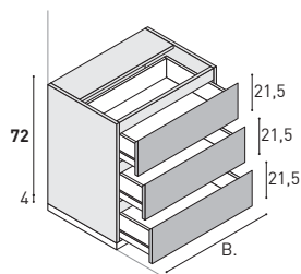
Unterschränk mit 3 Auszügen.
