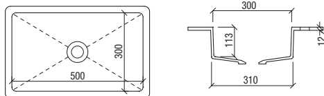
VENUS HPE1 50 x 30 cm für Waschtisch-Unterschranke ≥ 60
