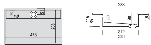
VEGA HPV1 47,8 x 28,8 cm für Waschtisch-Unterschranke ≥ 60
