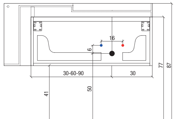
Waschtisch WRAP 2, Becken mit 1 Armaturenbohrung hinten mittig (Beispiel)
