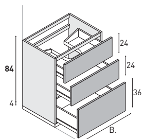
Waschtisch-Unterschrank mit 1 Auszüge H.36 + 2 Auszügen H.24.
