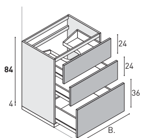
Waschtisch-Unterschrank mit 1 Auszüge H.36 + 2 Auszügen H.24.
