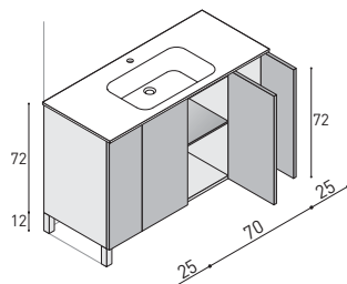
Waschtisch-Unterschrank mit 4 Türen, 3 Glas-Einlegeböden. Bodenstehend.
