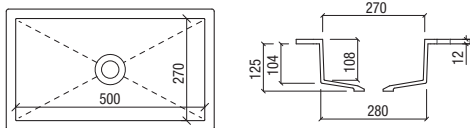
VENUS SMALL HPC1 50 x 27 cm für Waschtisch-Unterschranke ≥ 60
